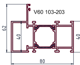
Усиленные профили
