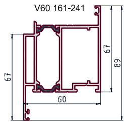
Цоколь
