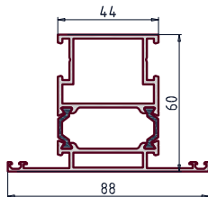
Импост
