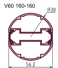
Поворотный профиль
