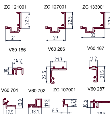
Доп. профиль
